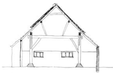
DOORSNEDEN OVER DE DEEL.
