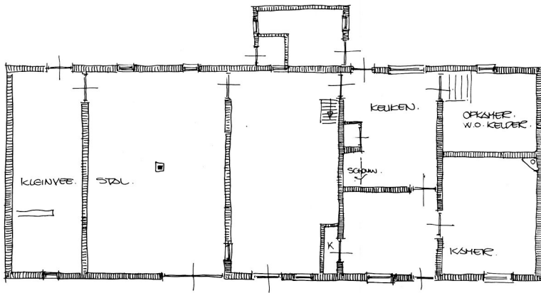
INDELING BEG.GROND.
